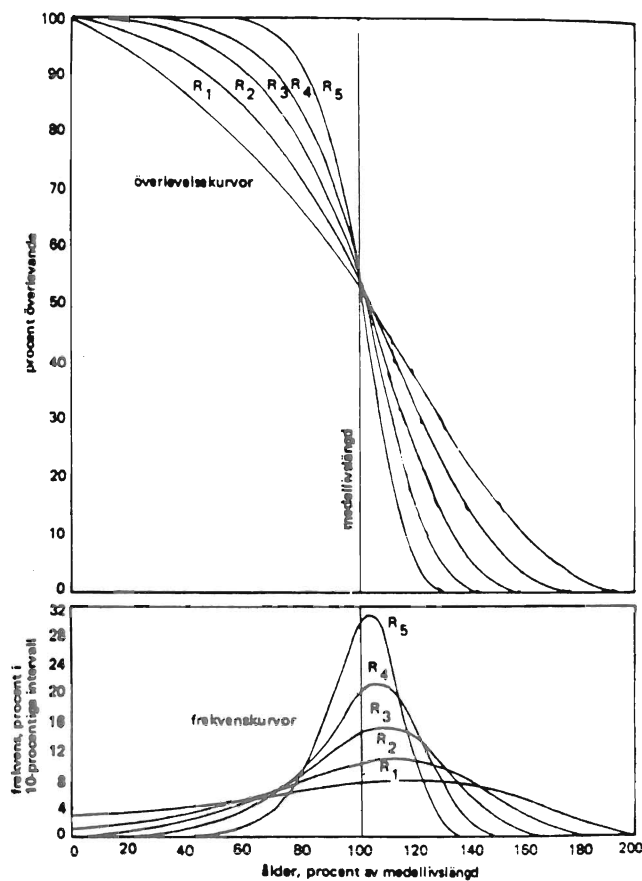
Figur 3: Högerskeva överlevelsekurvor.
